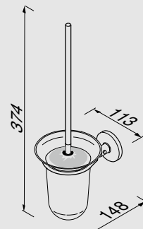
915311-02 Toiletborstelhouder, wandmodel Toiletbrush holder, wall mounted Porte-balai, fixation murale WC-Bürstengarnitur, zur Wandmontage Набор с ершиком для унитаза, отдельный
