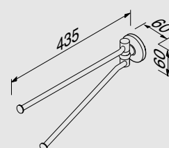
915305-02 2-lids handdoekhouder 2 arm Towel holder Porte serviettes, 2 barres Handtuchhalter 2-armig Полотенцедержатель, двойной
