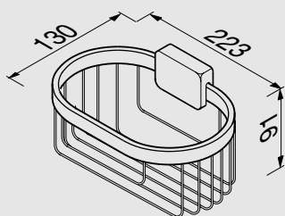
917014 Fles- en sponshouder Bottle/sponge holder Universalkorb Corbeille universelle Держатель бутылки/губки + полочка
