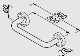
915531-30 Badgreep 30 cm Grab rail 30 cm Wannengriff 30 cm Poignée de bain 30 cm Поручень 30 см
