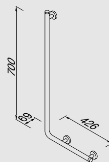
915808-02-L Veiligheidsgreep 90° Safety grip handle 90° Sicherheitsgriff 90° Poignée de sécurité 90° Поручень безопасности 90°
