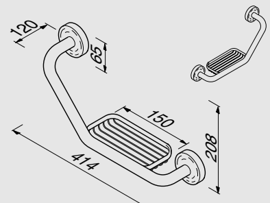
915528 Badgreep met zeephouder Grab rail with soap holder Wannengriff mit Seifenkorb Poignée de bain avec porte savon Поручень с мыльницей
