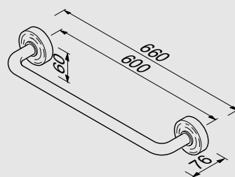
915531-60 Wandhanddoekhouder 60 cm Towel rail 60 cm Wandhandtuchhalter 60 cm Porte serviettes 60 cm Настенный полотенцедержатель 60 см
