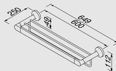
917352-04 Badhanddoekplateau 60 cm Bath towel shelf 60 cm Badetuchablage 60 cm Plateau pour serviettes de bain 60 cm Полка для полотенец 60 см
