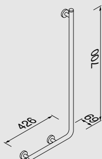
915808-02-R Veiligheidsgreep 90° Safety grip handle 90° Sicherheitsgriff 90° Poignée de sécurité 90° Поручень безопасности 90°
