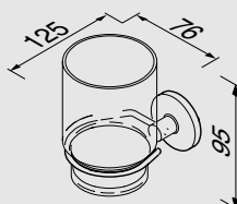
915302-02 Glashouder Tumbler holder Porte-verre Becherhalter держатель стакана
