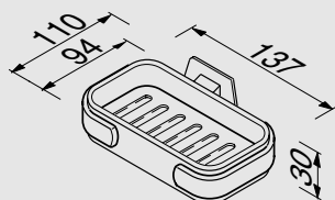
915155 Zeephouder met witte kunststof inzet Soap holder with white plastic tray Seifenhalter mit weisser Kunststoffeinsatz Porte-savon avec coupelle synthétique blanche Мыльница с пластиковой белой чашей
