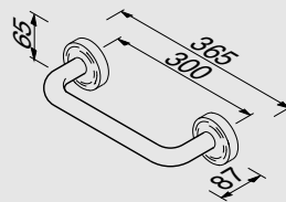
915529-30 Badgreep 30 cm Grab rail 30 cm Wannengriff 30 cm Poignée de bain 30 cm Поручень 30 см
