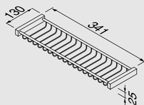
9112514-02-35 Fles- en sponshouder Bottle/sponge holder Universalkorb Corbeille universelle Держатель бутылки/губки + полочка
