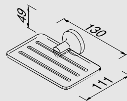
917343-02 Zeephouder Soap holder Seifenhalter Porte-savon Мыльница
