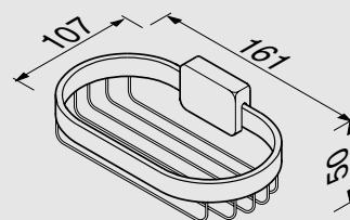
917006 Spons- en zeephouder Sponge/soap holder Kombikorb Porte-savon/éponge Мыльница/держатель губки
