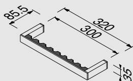
913506-02 Badgreep 30 cm Grab rail 30 cm Wannengriff 30 cm Poignée de bain 30 cm Поручень 30 см
